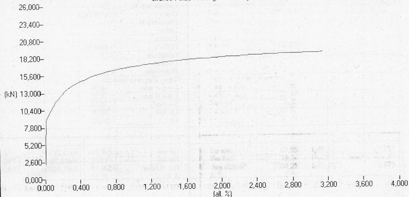
Grafico Forza / Allungamento (Traversa)
